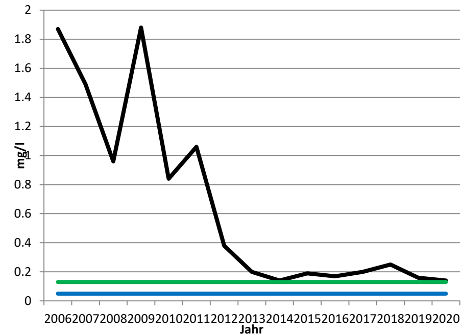
Jahresdurchschnittskonzentrationen von Ammonium an der Station ALZETTE-Ettelbruck von 2006-2020
