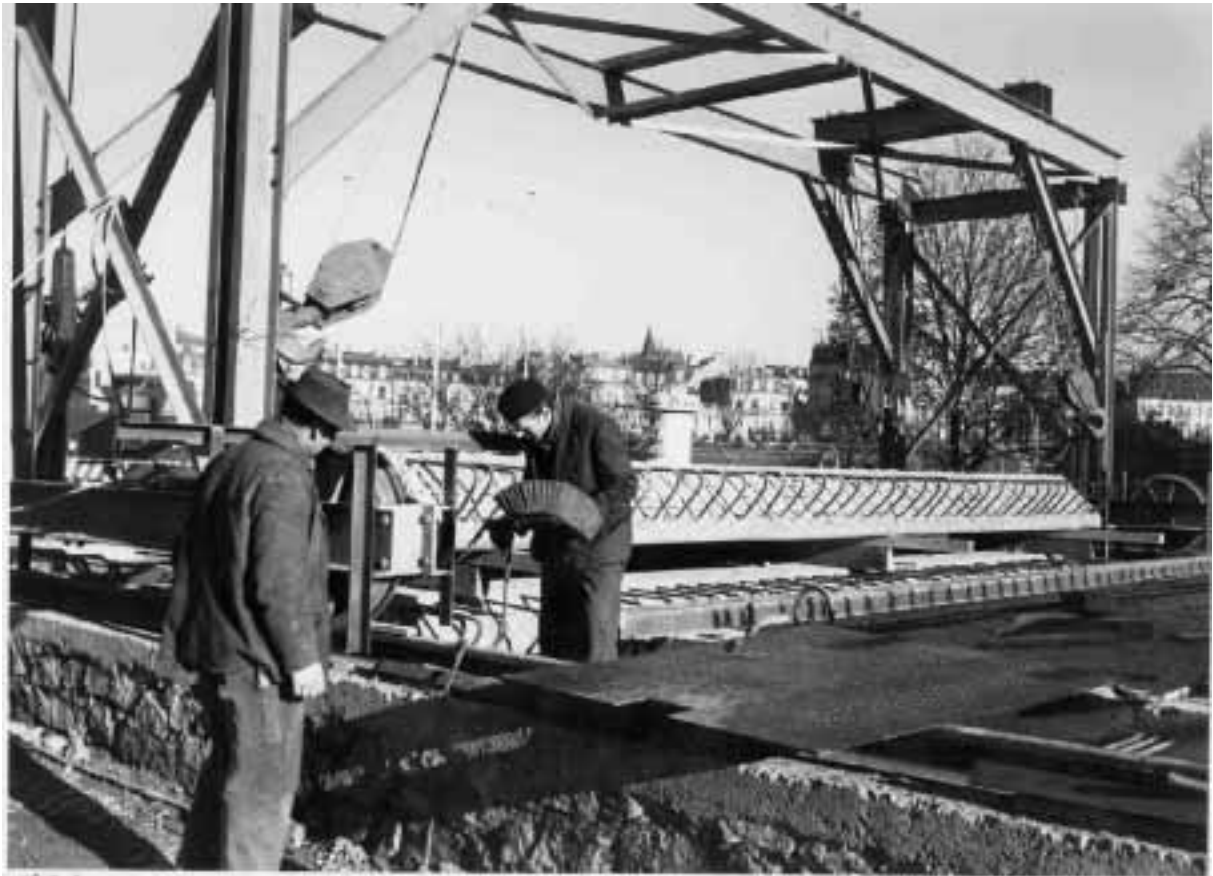
Le renouvellement du tablier en 1961/62
