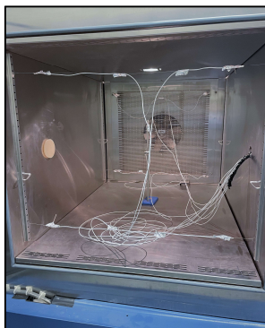
Photo: Caractérisation d'une enceinte thermique
