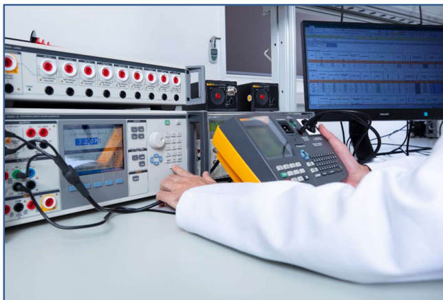
Photo: Étalonnage d'un testeur électrique
