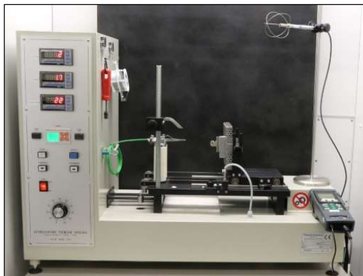
Photo: Équipement Glow-Wire
